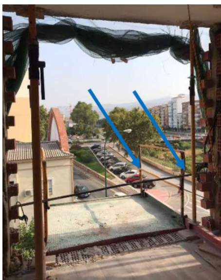
Vista del montacargas montado tras el accidente. El operario cayó al vacío desde la tercera planta del edificio junto con la plataforma de carga, debido a su insuficiente enclavamiento en la edificación.
