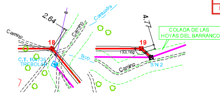
PLANTA
