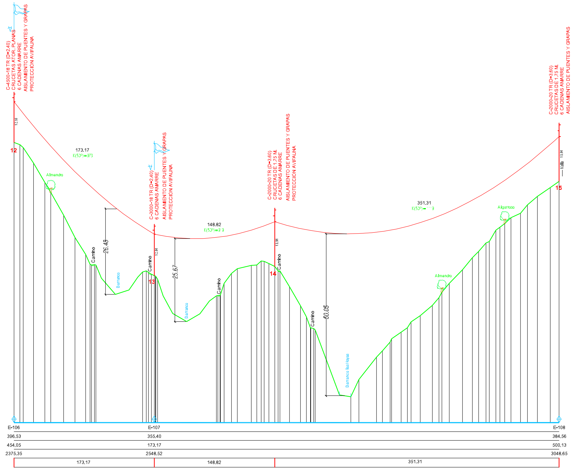
PERFIL
