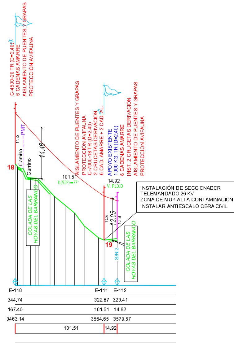
PERFIL
