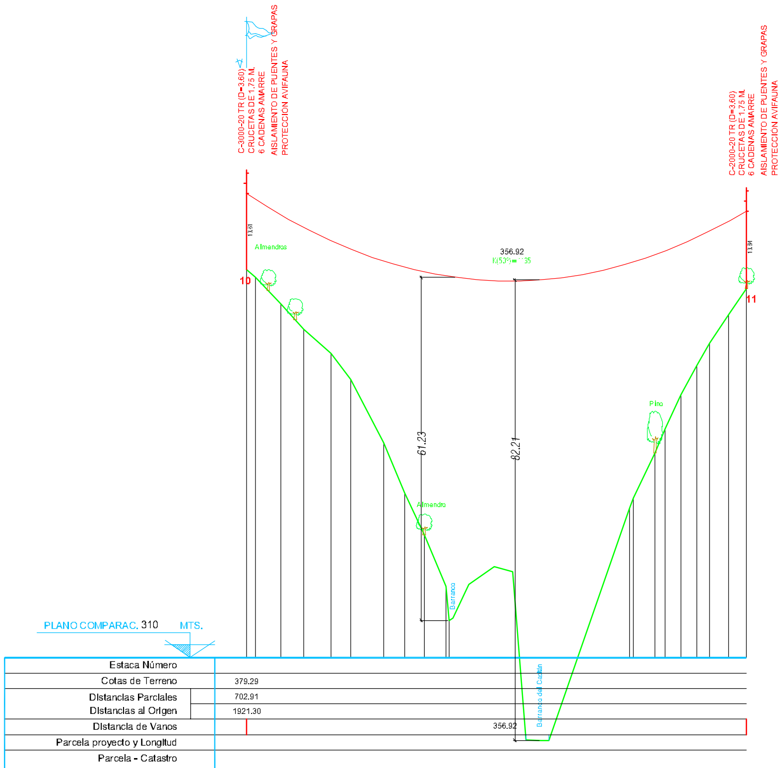
PERFIL
