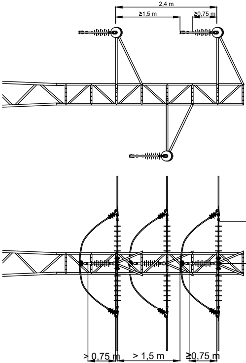
MEDIDAS ANTI-ELECTROCUCCION AVIFAUNA
