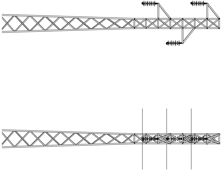
MEDIDAS ANTELECTROCUCIÓN AVIFAUNA
