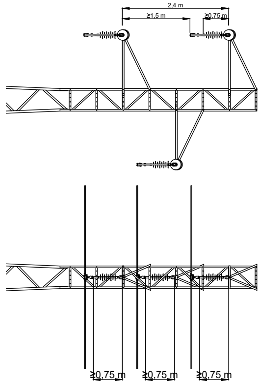
MEDIDAS ANTELECTROCUCIÓN AVIFAUNA
