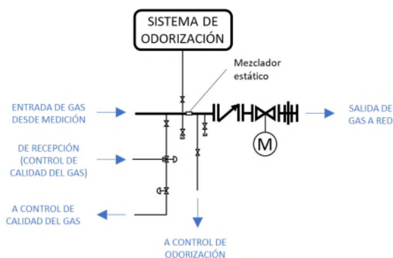
Imagen 3: Esquema orientativo del sistema de odorización y salida de gas aceptado.
