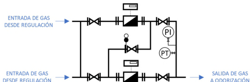
Imagen 2: Esquema de instalación mecánica del bloque de medida de gas aceptado.
