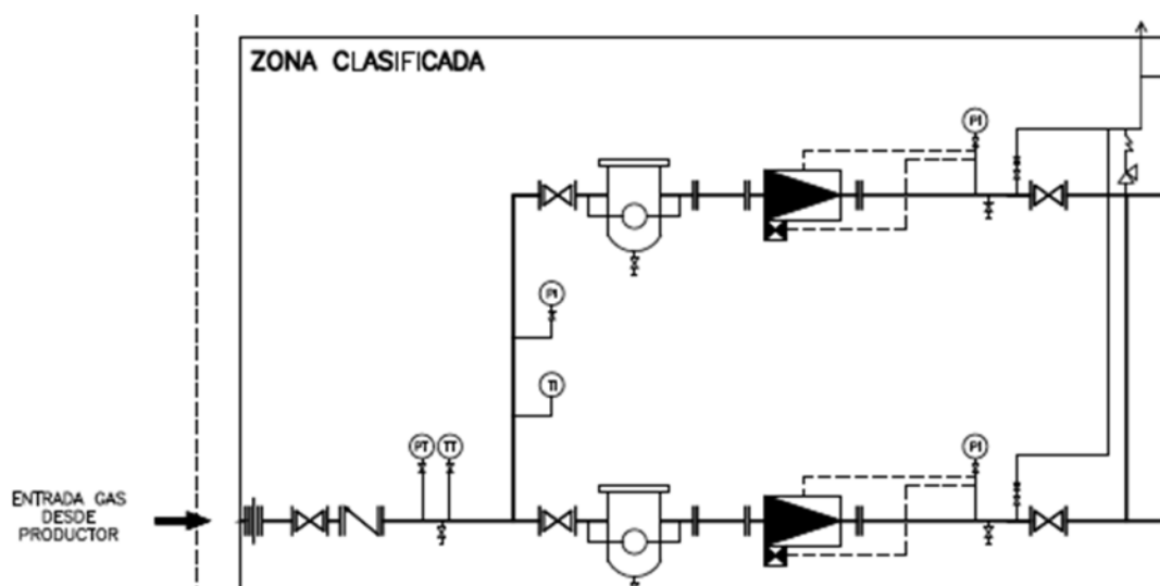
Imagen 1: Esquema orientativo de instalación mecánica del bloque de filtrado y regulación de gas aceptado.
