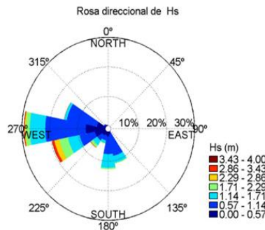
Figura 10. Oleaje en la UC-CA13. Fuente: Estrategias para la protección costera en las provincias de Cádiz, Málaga y Almería considerando los efectos del cambio climático. Anejo 1. Caracterización del clima marítimo. 2019.
