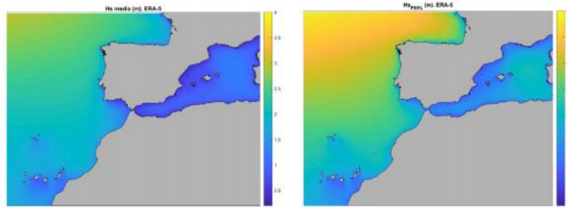
Figura 8. Valores medios (izquierda) y percentil del 99% de la altura de ola significativa (m) (derecha), obtenidos a partir de las variables atmosféricas procedentes del reanálisis ERAS (1985-2005). Fuente: Estrategia española para la adaptación de la costa al cambio climático.
