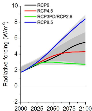
Figura 1. Forzamiento radiativo de las vías de concentración representativas. El área gris claro captura el 98% del rango en escenarios IAM anteriores, y el gris oscuro representa el 90% del rango. Fuente: Web IPCC. De van Vuuren et al (2011) The Representative Concentration Pathways: An Overview. Cambio climático, 109 (1-2), 5-31.
