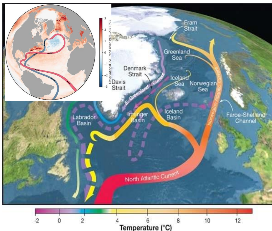
Figura 13. Flujos superficiales actuales (líneas continuas) y los flujos profundos (líneas discontinuas) para el Atlántico norte y los mares nórdicos. Figure modified from R. Curry and C. Mauritzen © Woods Hole Oceanographic Institution. Disponible en: https://tos.org/oceanography/article/is-the-atlantic-overturing-circulation-approaching-a-tipping-point
