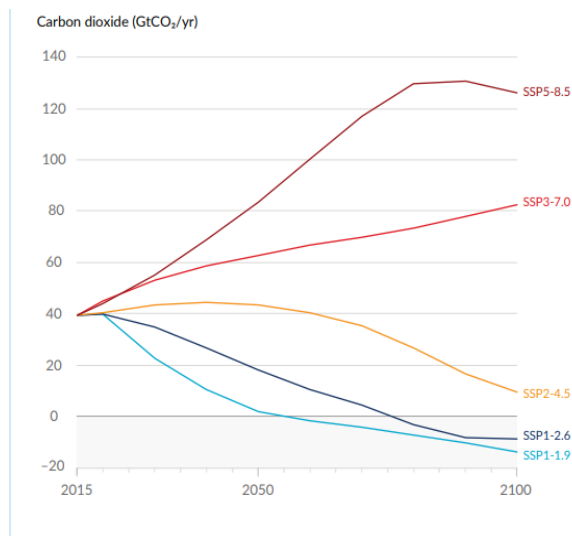
Figura 3. Sendas representativas de emisiones según AR6. Fuente: Resumen para los formuladores de políticas. Cambio Climático 2021: La Base de la Ciencia Física. Contribución GTI al Sexto Informe IPCC 7
