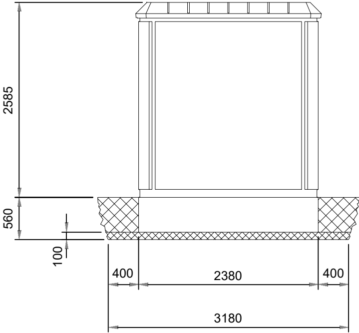
VISTA LATERAL
