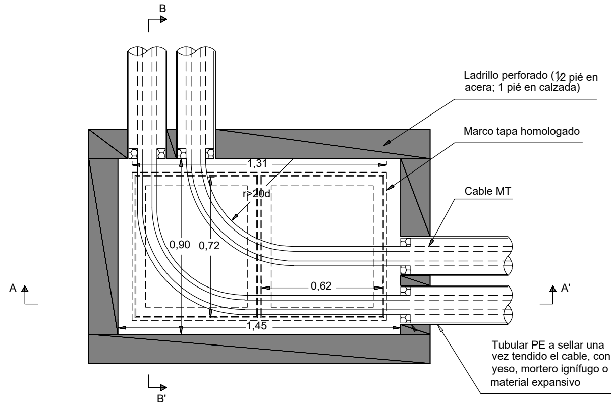
PLANTA
