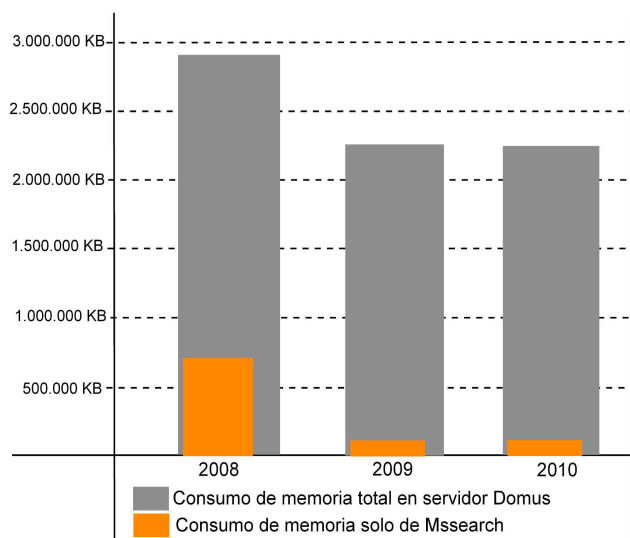
GRÁFICO 4. COMPARATIVA DE CONSUMO DE MEMORIA DOMUS-SERVICIO MSSEARCH
