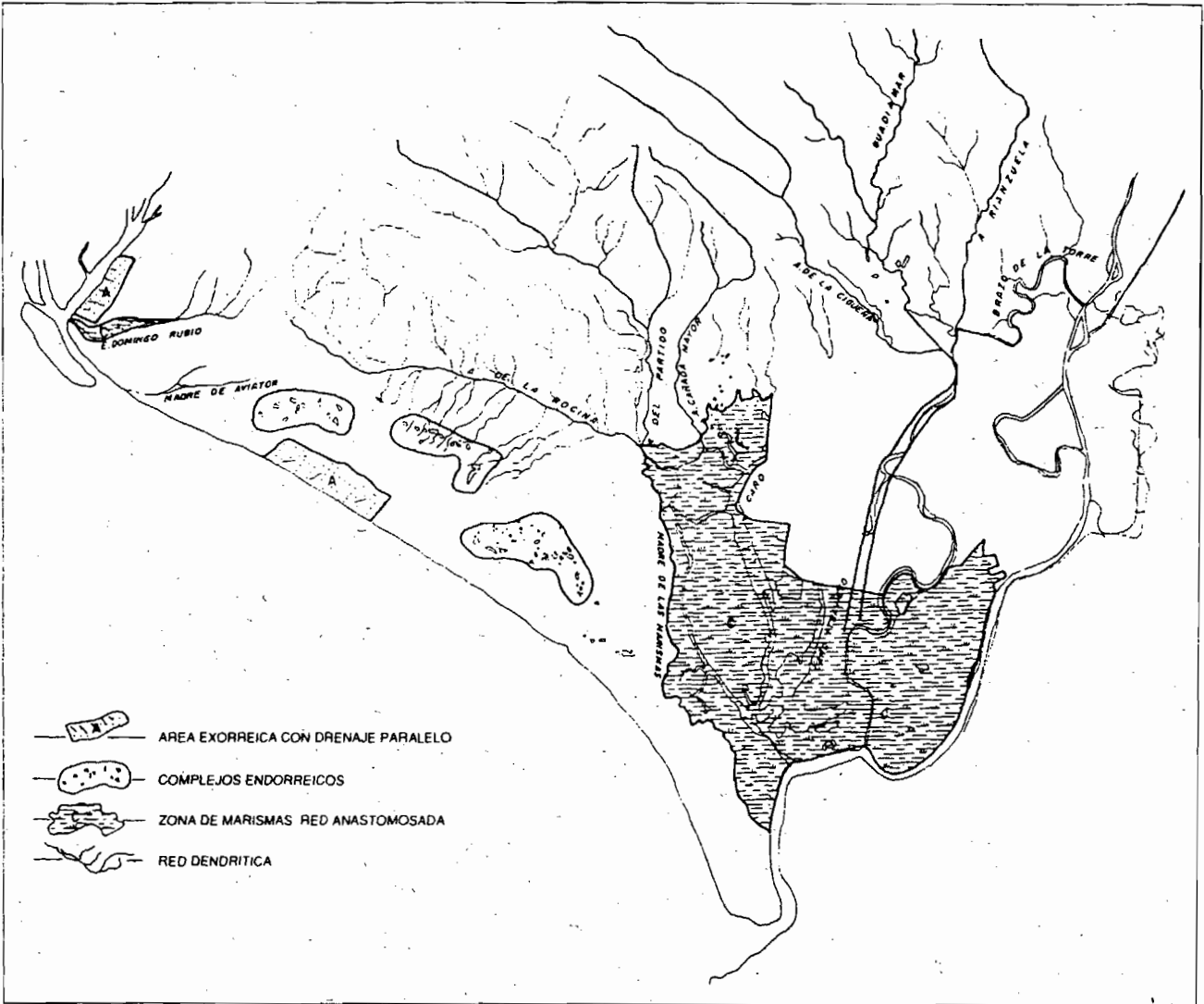
Mapa 6. REDES DE DRENAJE
